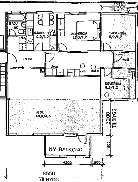
PLAN 2. ETASJE UTBYGGET LEILIGHET
