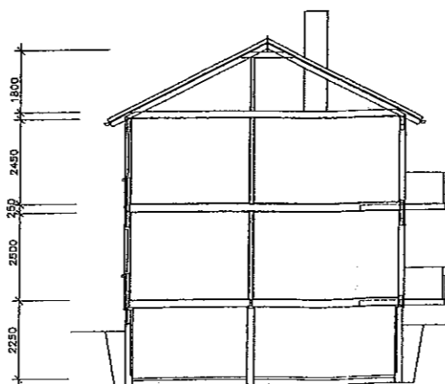
SNITT (opprinnelig bygn.)
