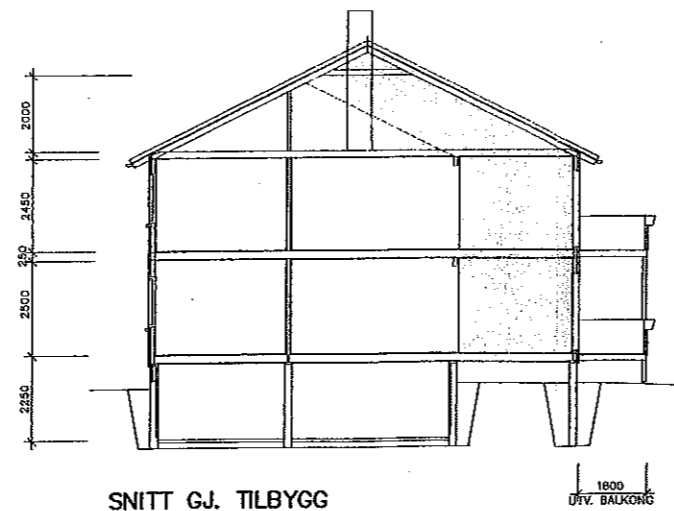
SNITT GJ. TILBYGG
