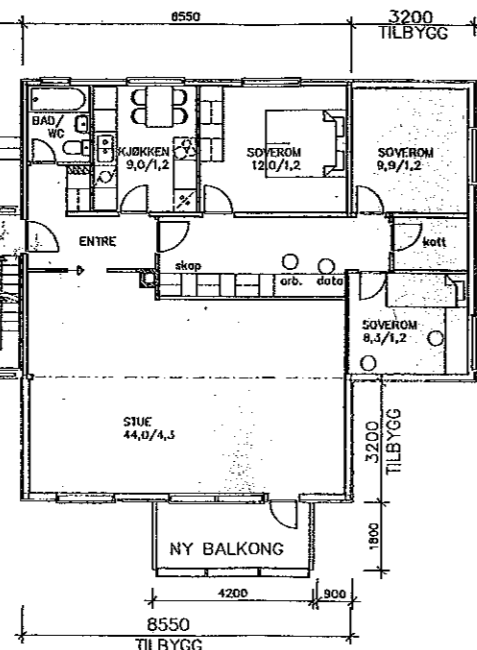
PLAN 1. ETASJE UTBYGGET LEILIGHET
