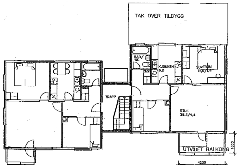
PLAN 2. ETASJE UTVIDET BALKONG
