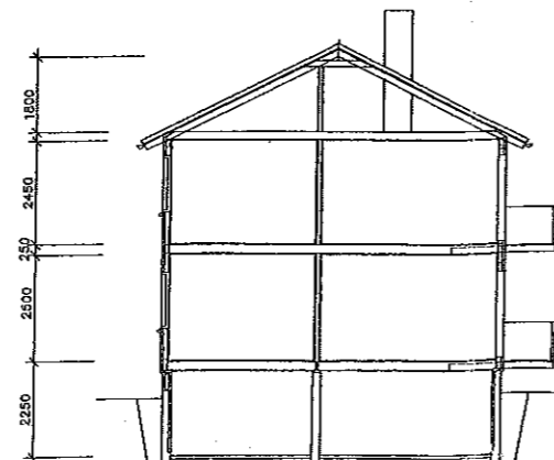
SNITT
