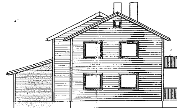
GAVL NORD-VEST
