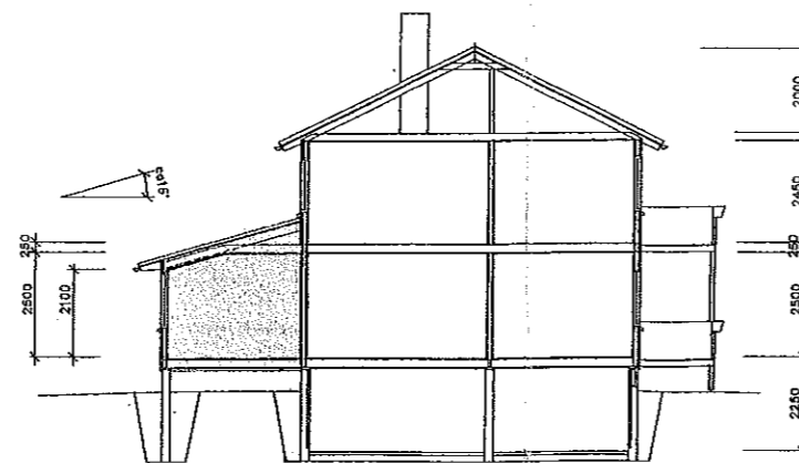
SNITT G.J. TILBYGG
