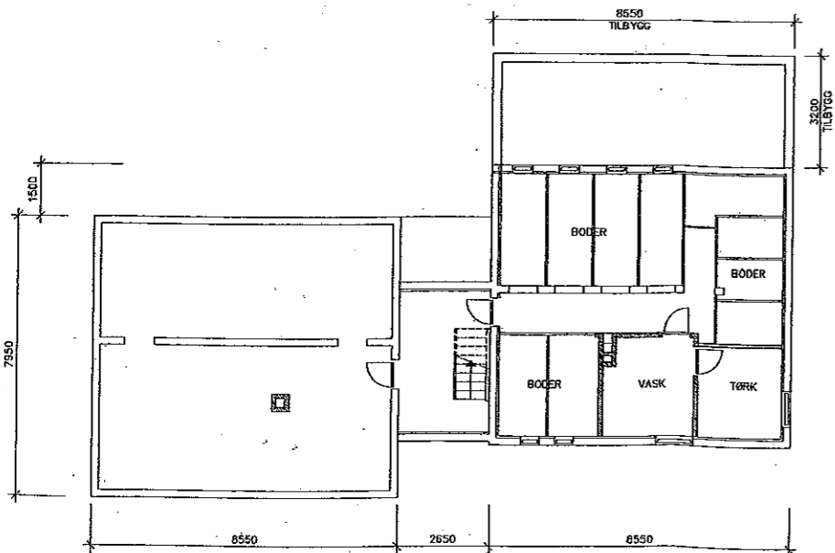
PLAN KJELLER
