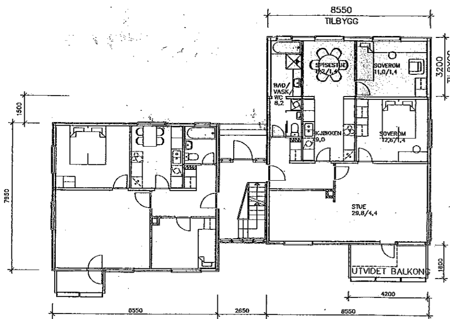
PLAN 1. ETASJE OPPRINNELIG SITUASJON
