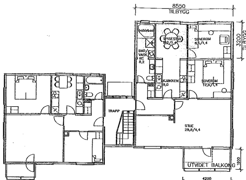
PLAN 2. ETASJE OPPRINNELIG SITUASJON
