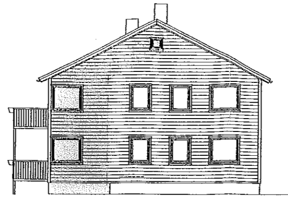
GAVL SYD-ØST UTBYGGET LEILIGHET
