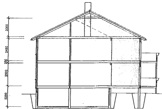
SNITT GJ. TILBYGG
