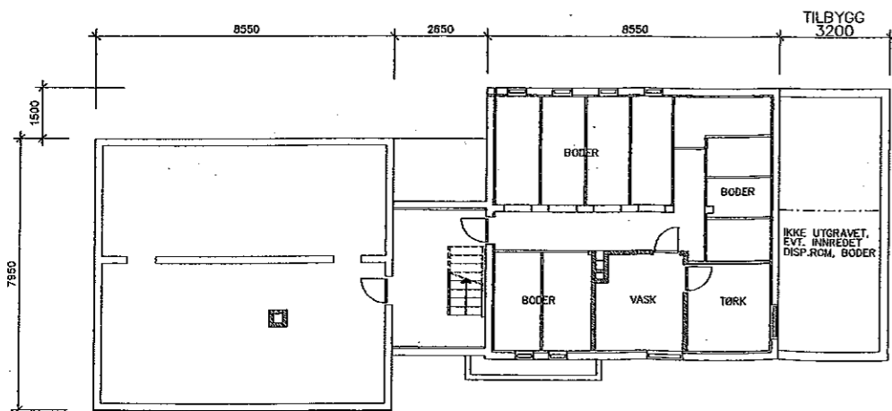
PLAN KJELLER
