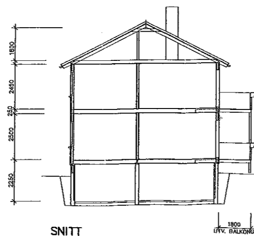
SNITT
